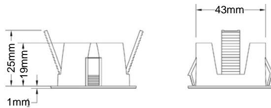
Flush ring
